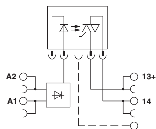
Электрическая схема
