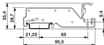
Размерный чертеж
