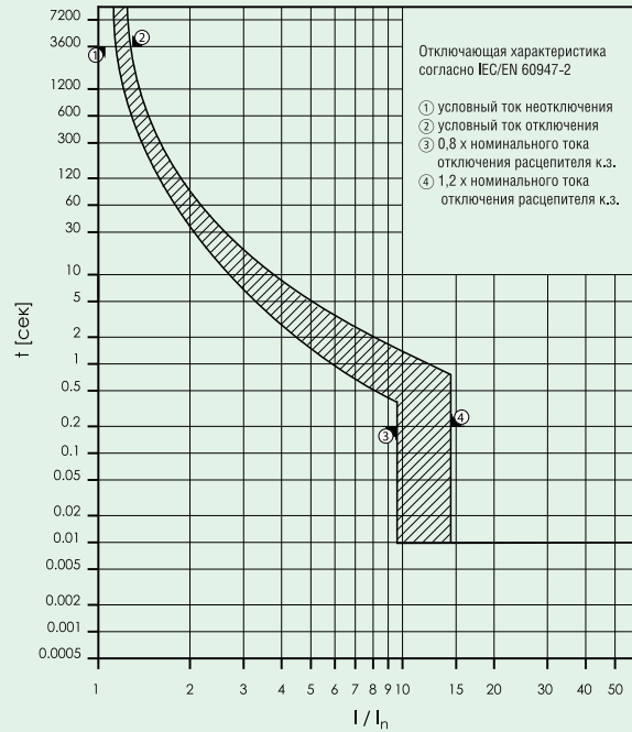
Кривая отключения BZM1 80A, 3-х полюсное исполнение
