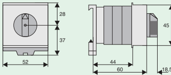
Размеры [мм]
