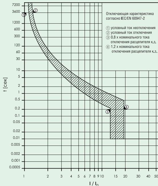
Кривая отключения BZM1 32A, 3-х полюсное исполнение
