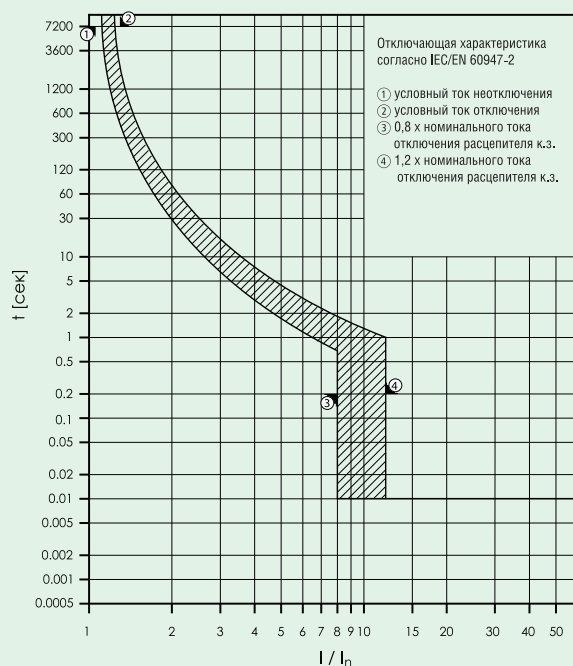
Кривая отключения BZM1 100A, 3-х полюсное исполнение
