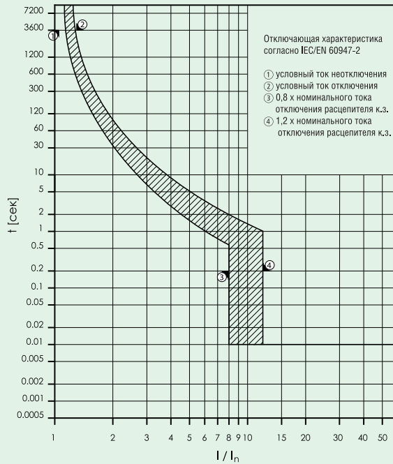
Кривая отключения BZM1 63A, 3-х полюсное исполнение
