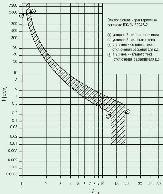
Кривая отключения BZM1 25A, 3-х полюсное исполнение
