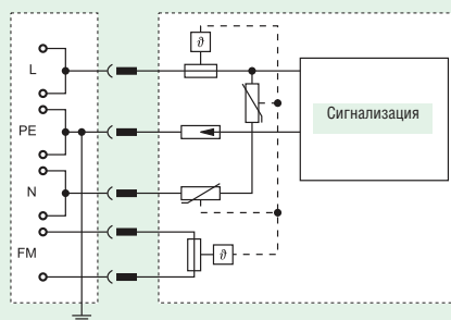
Схема соединения
