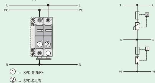
Схема соединения
