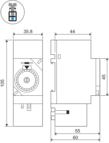
12.21 Винтовой зажим
