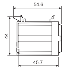
062.08 с реле
