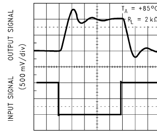
TIME (1 \mu s /div) DS012830-26
