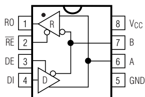
DIP/SO
