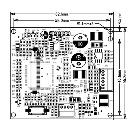
Рис.3 Установочные размеры
