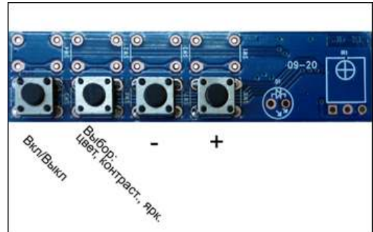
Рис.2 Назначение кнопок на плате управления.
