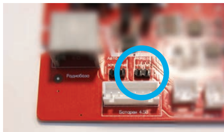
Минимальная чувствительность – перемычка удалена
