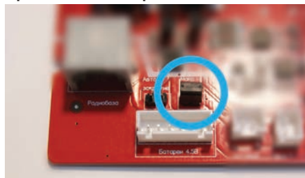
Максимальная чувствительность – перемычка установлена
