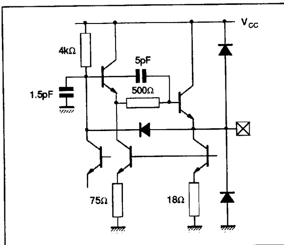
Pin : VIN
