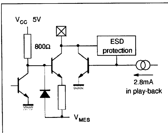
Pin : Iout
