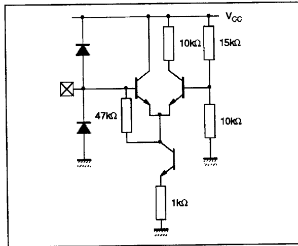
Pin : VMES
