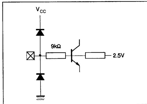
Pin : VREC
