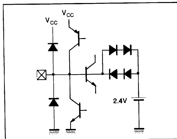
Pin : CAGC
