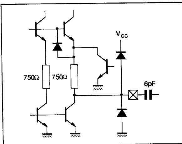
Pin : VIN
