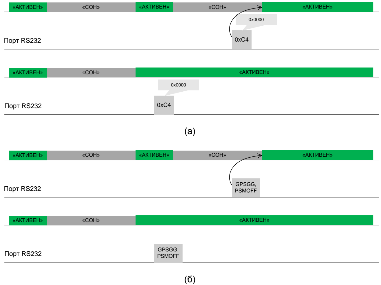
Рис. 21. Временные диаграммы выхода из режима RELAXED FIX®: (а) используя «0xC4»; (б) используя $GPSGG,PSMOFF
