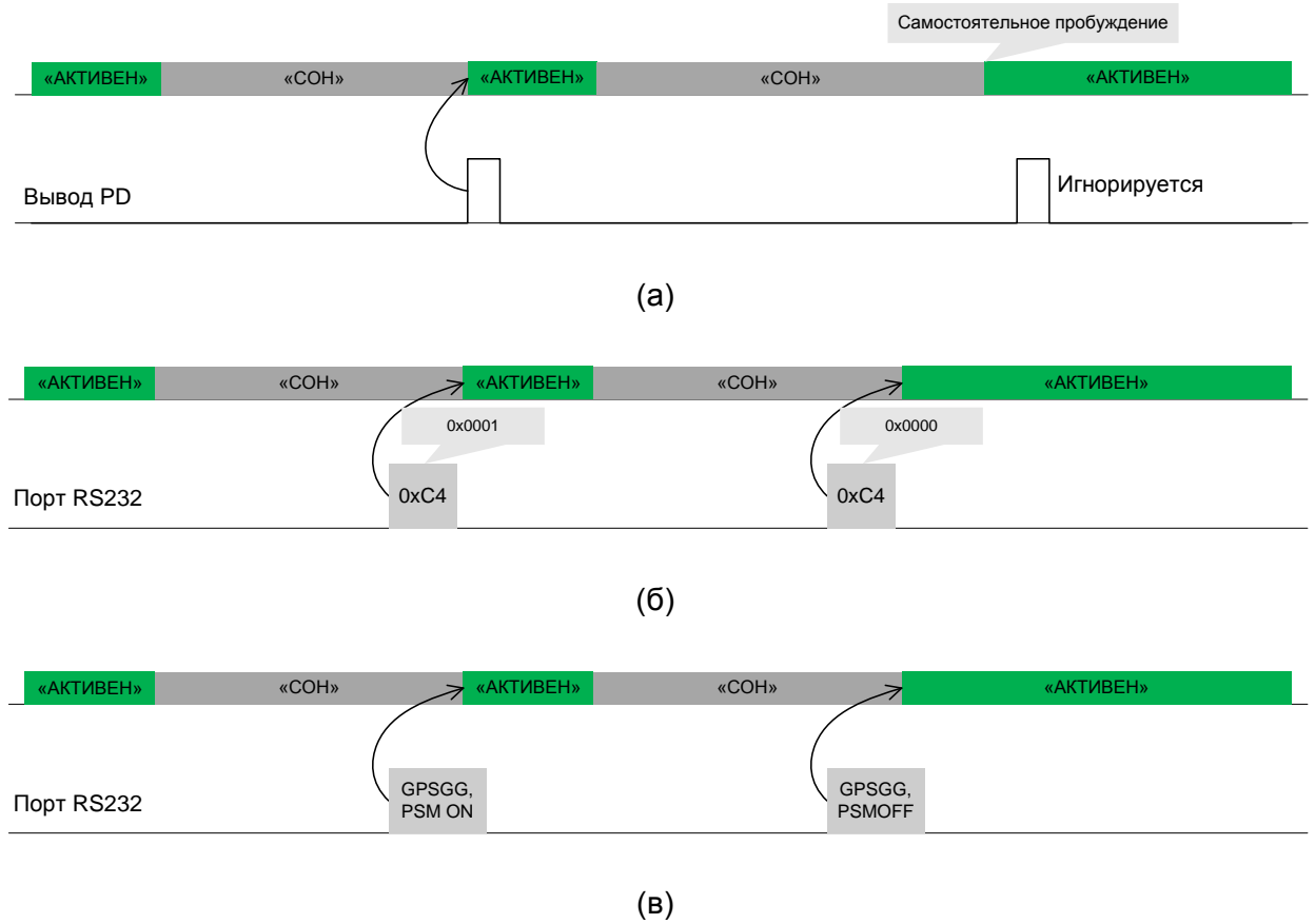
Рис. 22. Временные диаграммы пробуждения и выхода из режима FIX-BY-REQUEST®: (а) пробуждение выводом PD и самостоятельное пробуждение; (в) пробуждение, используя «0xC4»: 0x0001, и пробуждение/выход из режима, используя «0xC4»: 0x0000; (в) пробуждение, используя $GPSGG,PSM ON, и пробуждение/выход из режима, используя $GPSGG,PSMOFF
