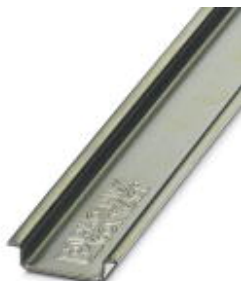
DIN-рейка, материал: сталь, без отверстий, высота 7,5 мм, ширина 35 мм, длина: 2 м
