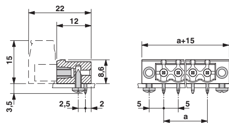
Размерный чертеж
