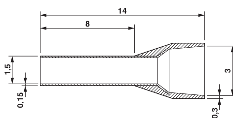
Размерный чертеж
