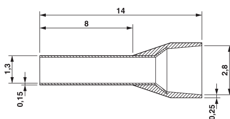
Размерный чертёж
