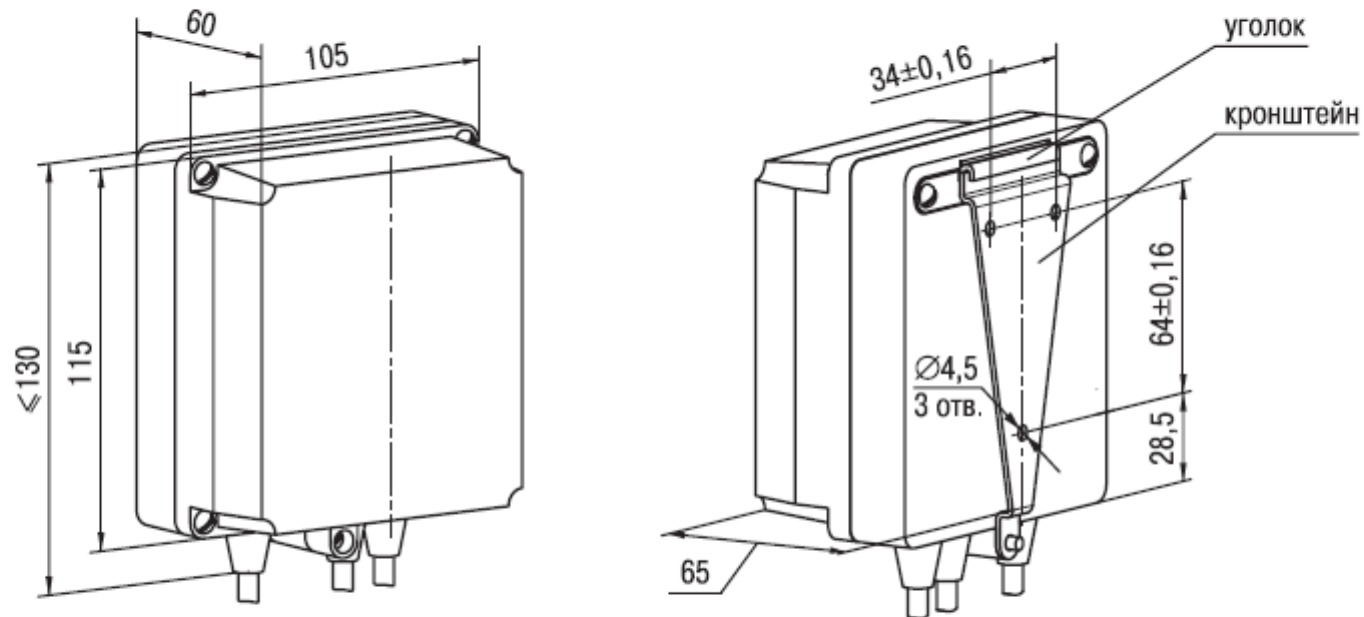
Рис. А.1. Корпус настенного крепления типа Н
