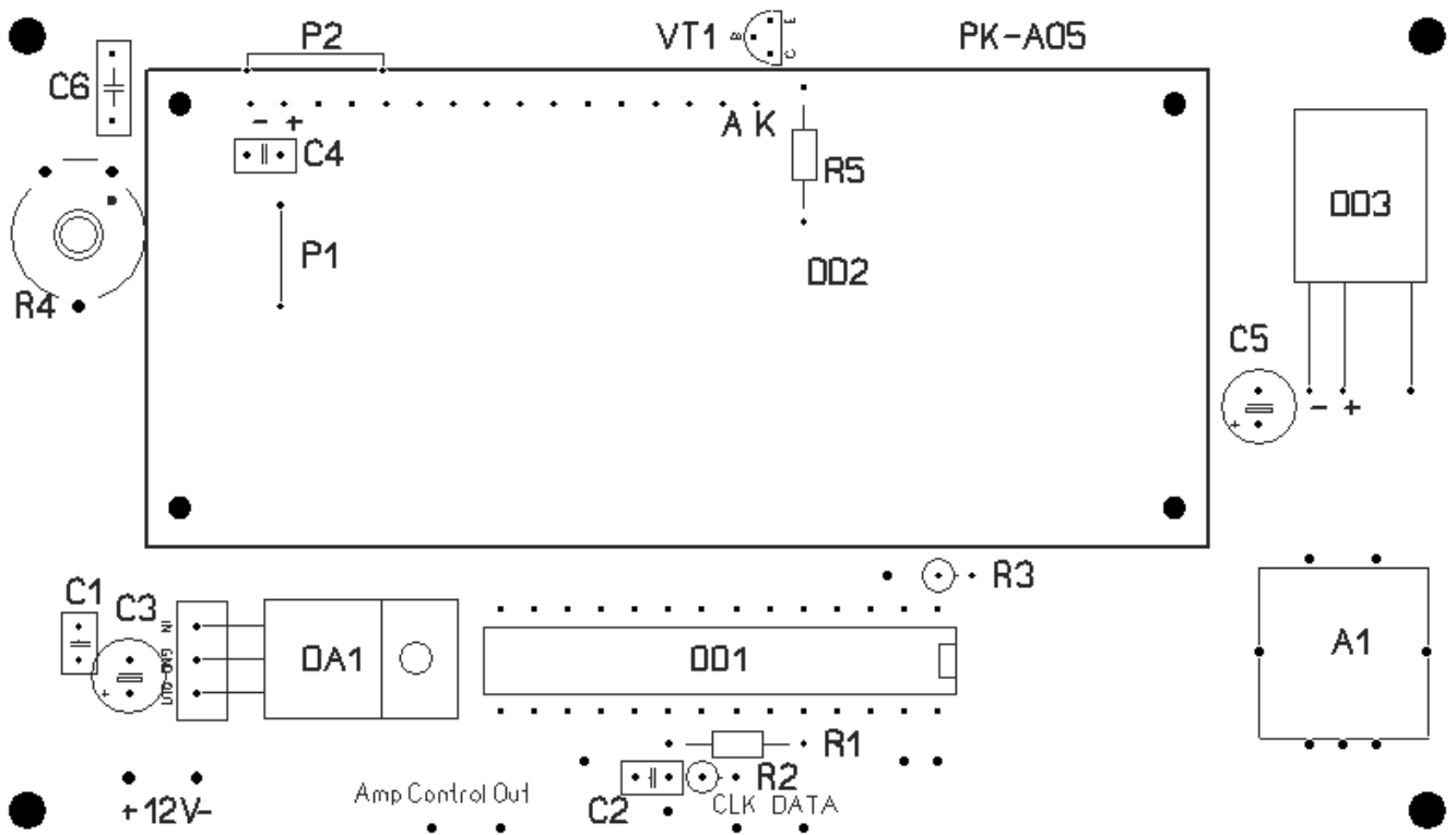
Рис. 3 Схема монтажная блока управления
