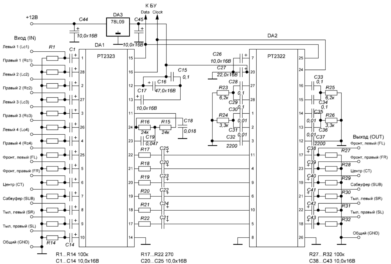
Рис. 1 Схема принципиальная блока управления
