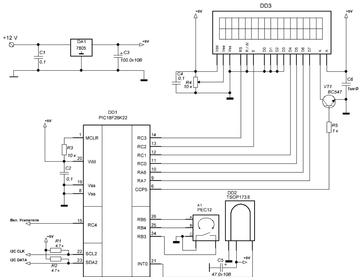
Рис. 1 Схема принципиальная блока управления
