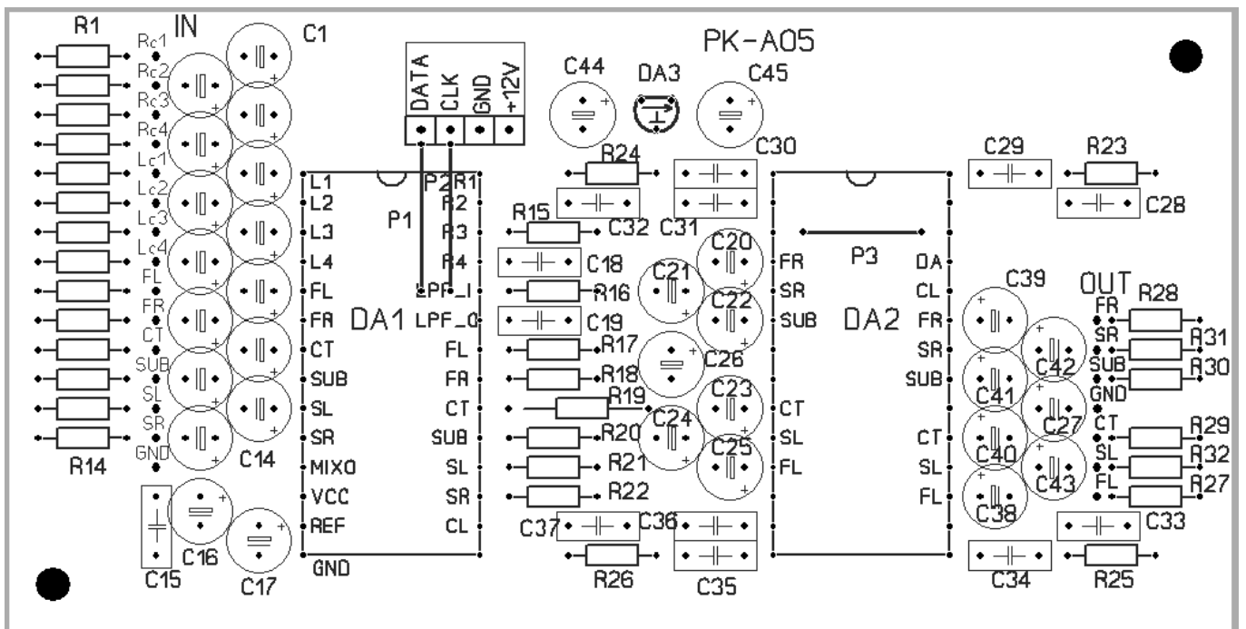
Рис. 4 Схема монтажная блока обработки сигнала
