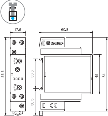
80.01 Винтовой зажим
