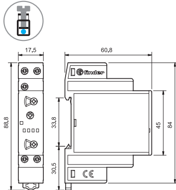
80.71 Винтовой зажим
