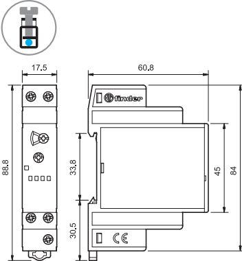
80.21 Винтовой зажим
