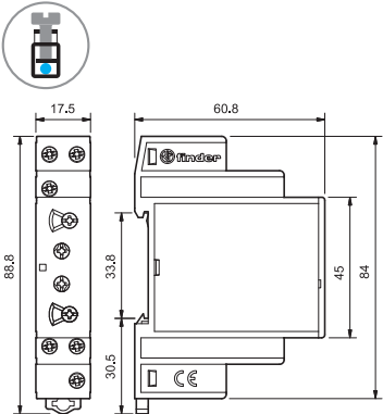
80.91 Винтовой зажим
