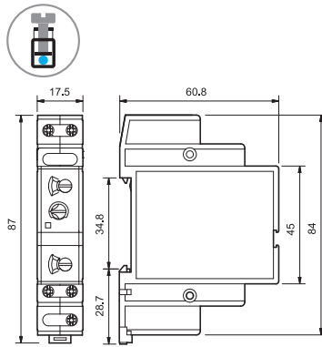
80.82 Винтовой зажим
