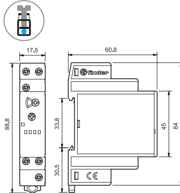
80.41 Винтовой зажим
