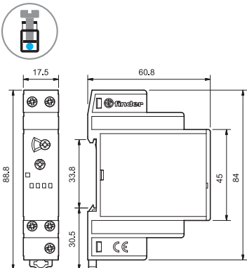
80.61 Винтовой зажим
