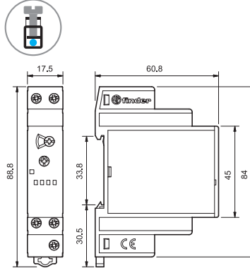
80.11 Винтовой зажим
