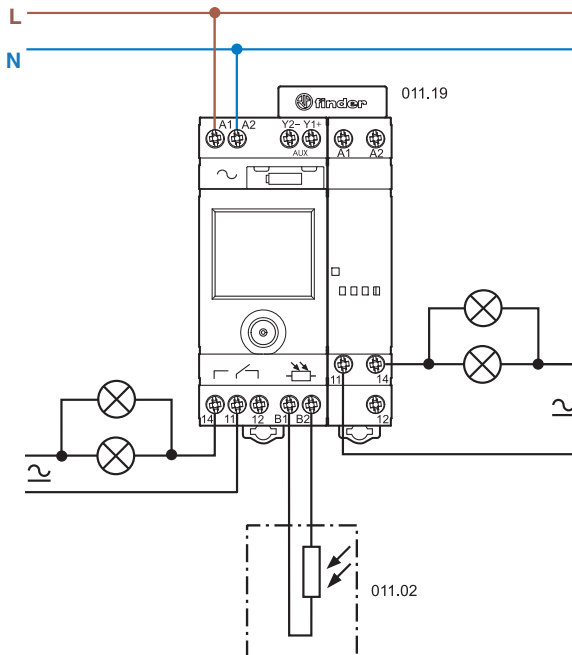
Тип 11.91 + 19.91
