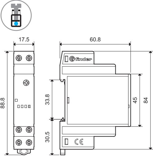
11.31 Винтовой зажим
