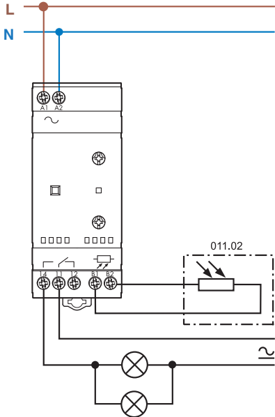
Тип 11.91 + 19.91
