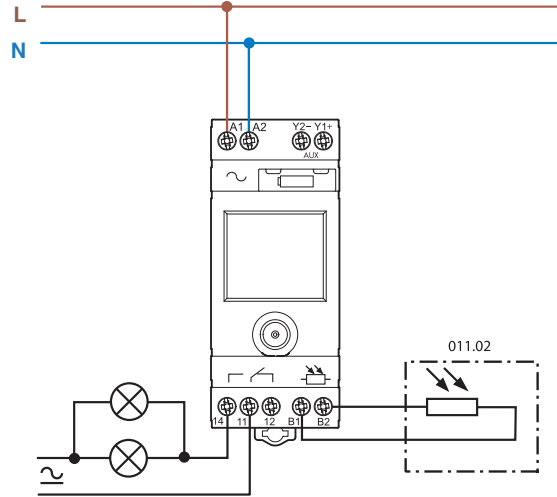
Тип 11.91
