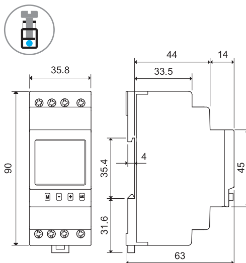
12.51/12.81 Винтовой зажим
