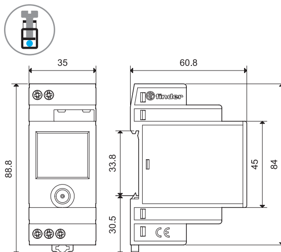
12.51/12.81 Винтовой зажим
