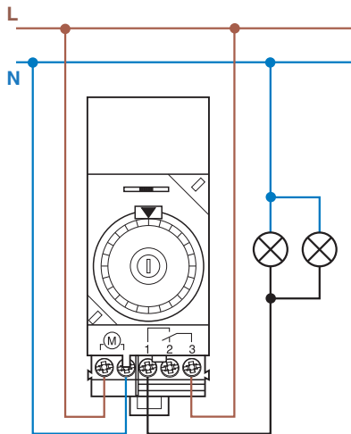
Тип 12.01 Селекторный переключатель: Ø = Постоянно ВЫКЛ AUTO = Авто I = Постоянно ВКЛ
