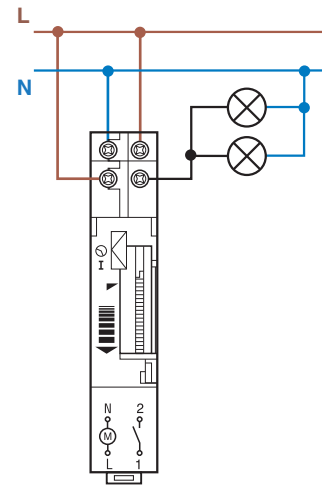
Тип 12.11 Селекторный переключатель: Ø = Авто I = Постоянно ВКЛ
