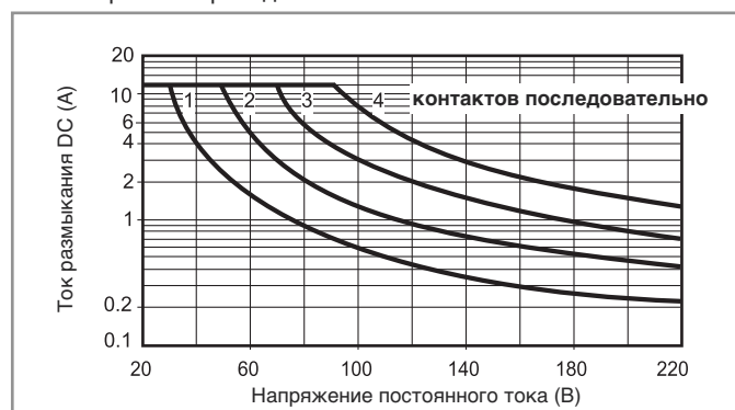
Н 56 - Макс. отключающая способность DC1 Версия с перекидным контактом
