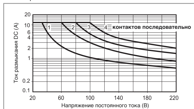
Н 56 - Макс. отключающая способность DC1 Версия с НО контактом
