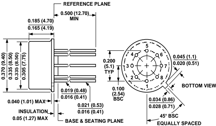
TO-99 (H-08A)
