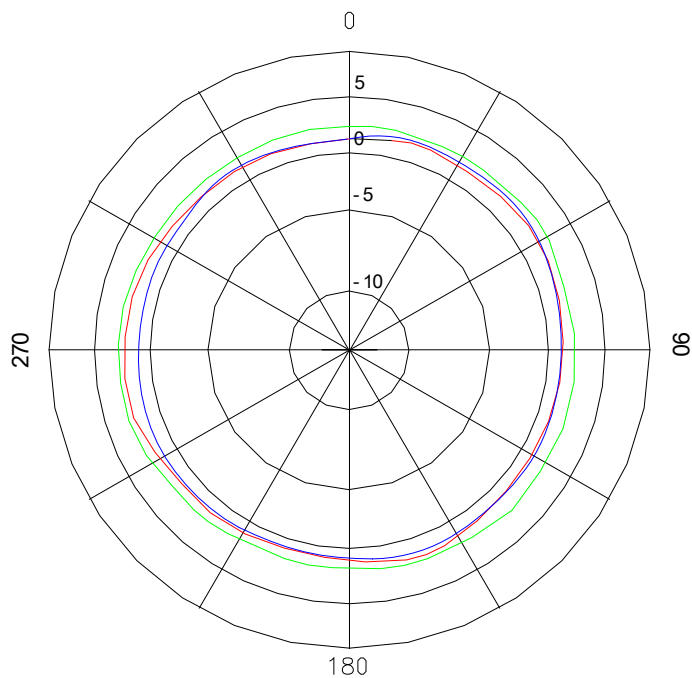
水平面方向图(2.4G天线) Horizontal Pattern
