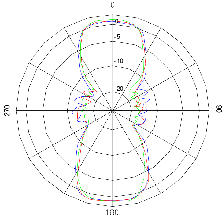
垂直面方向图 Vertical Pattern
