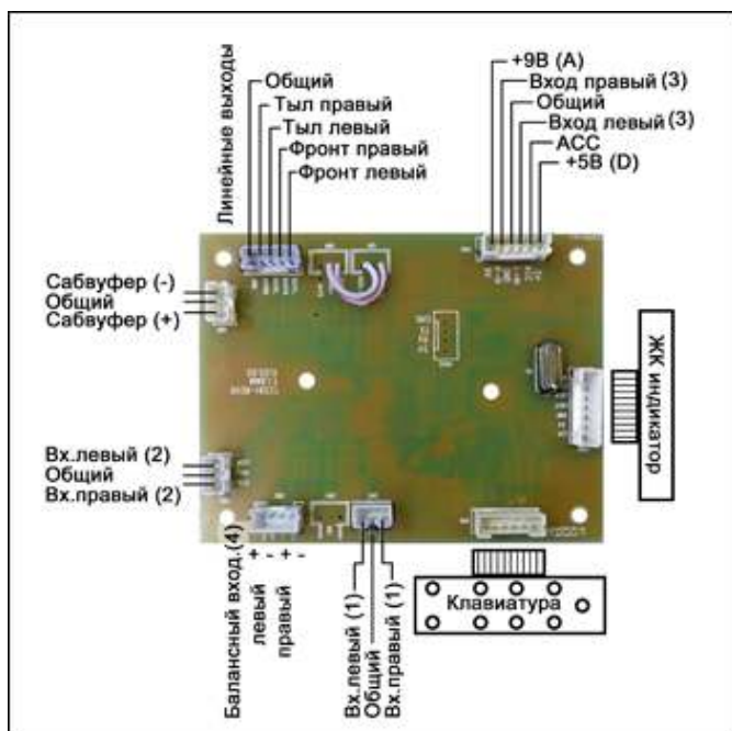
Рис.7 Схема подключения.
