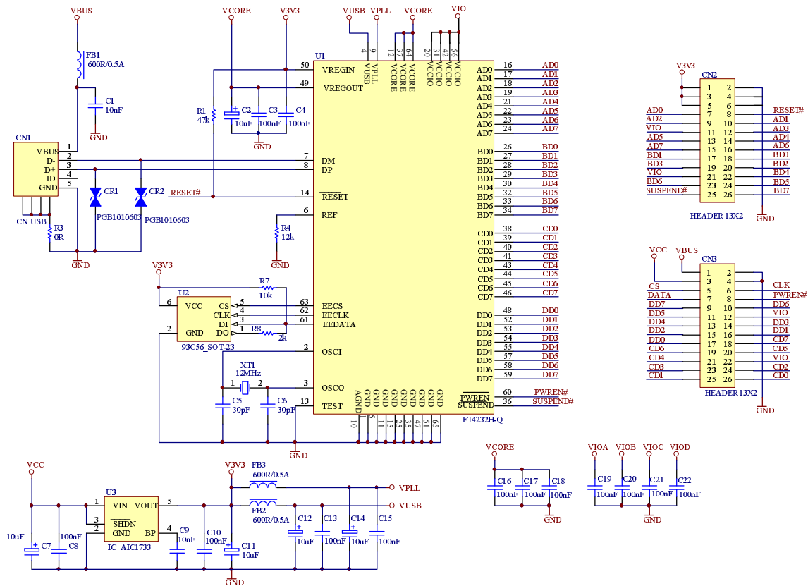
Figure 5.1 FT4232H Mini Module Schematic
