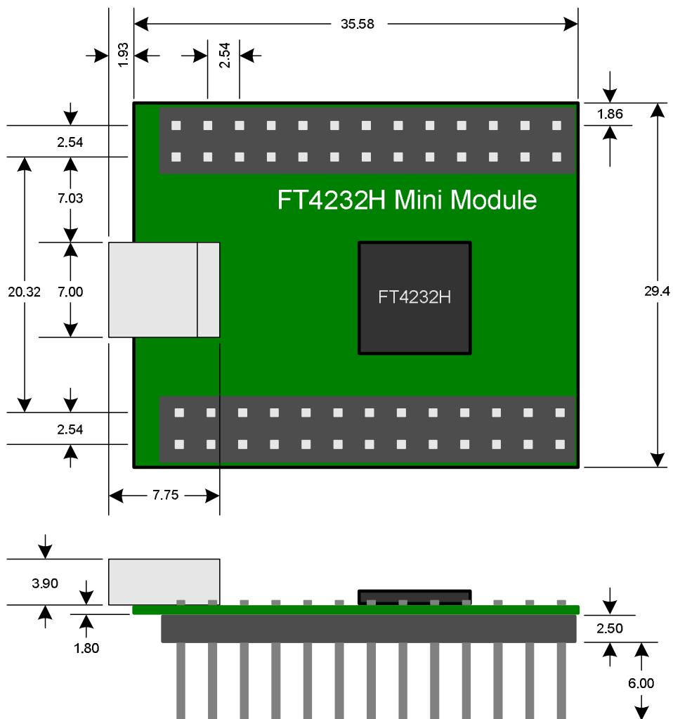
Figure 4.1 FT4232H Mini Module Dimensions
