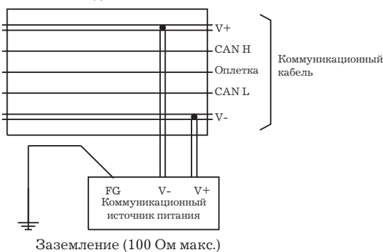
Разветвитель для источника питания
