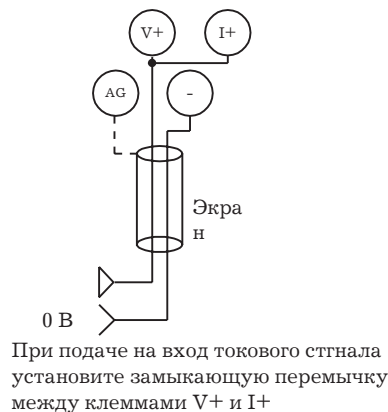
Вход по току
