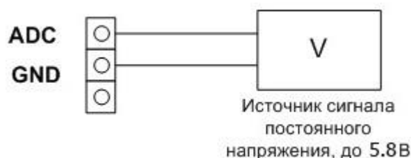
Рис. Схема подключения источника сигнала к АЦП
