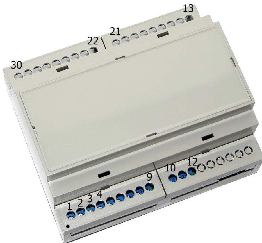
Рис.6.1 Расположение и наименование клеммных разъемов модуля
