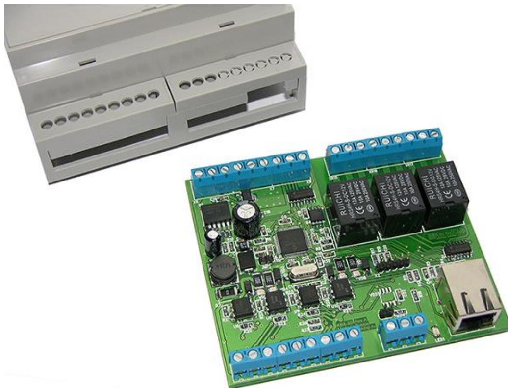
Рис.2. Плата модуля KBX-3D (без корпуса)
