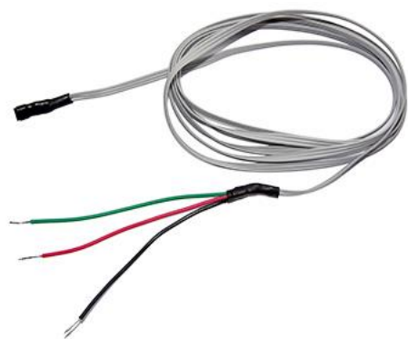
Рис. Датчик температуры KTS-18B20
