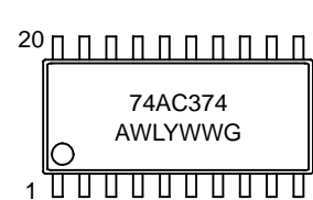
SOEIAJ–20
