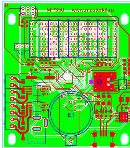
Рис. 4. Печатная плата.
