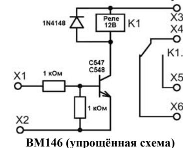
Рис.3. Схема подключения датчиков и других устройств.
