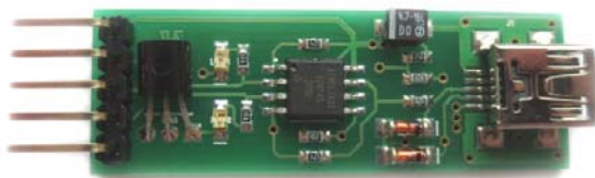
Рис.1. Общий вид устройства (показано без защитной термоусадочной трубки)
