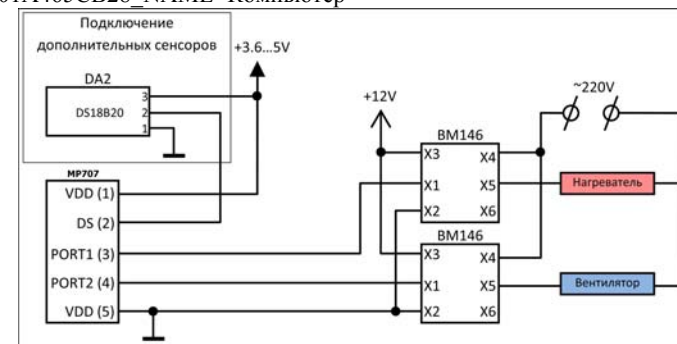
Рис.2. Подключение дополнительных устройств.
