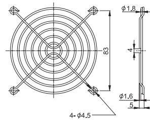
FG-09 For 92mm Fan
