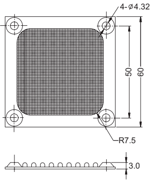
FM 06 For 60mm Fan
