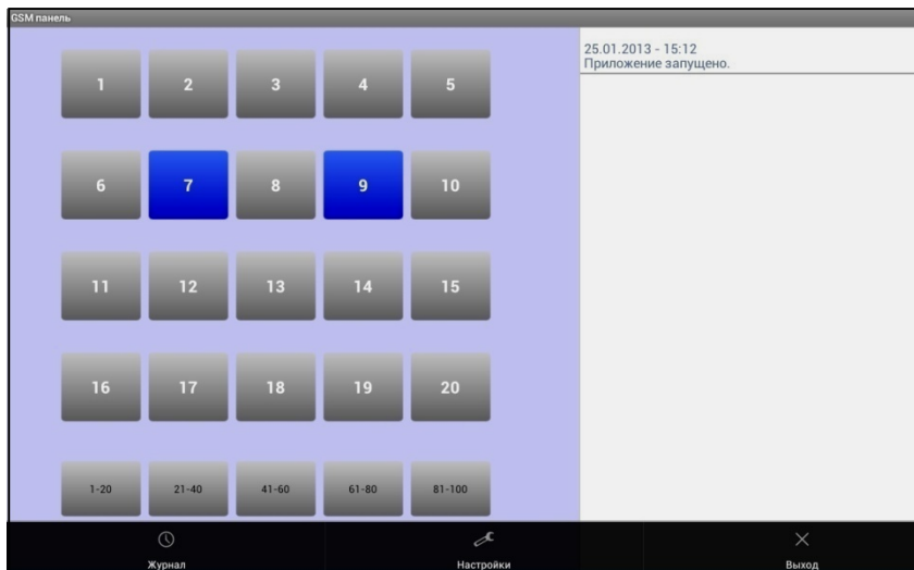
Рис.14 Окно программы
