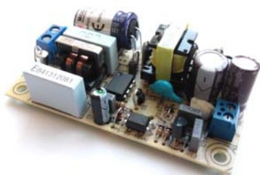
Общий вид устройства. Рис.1
