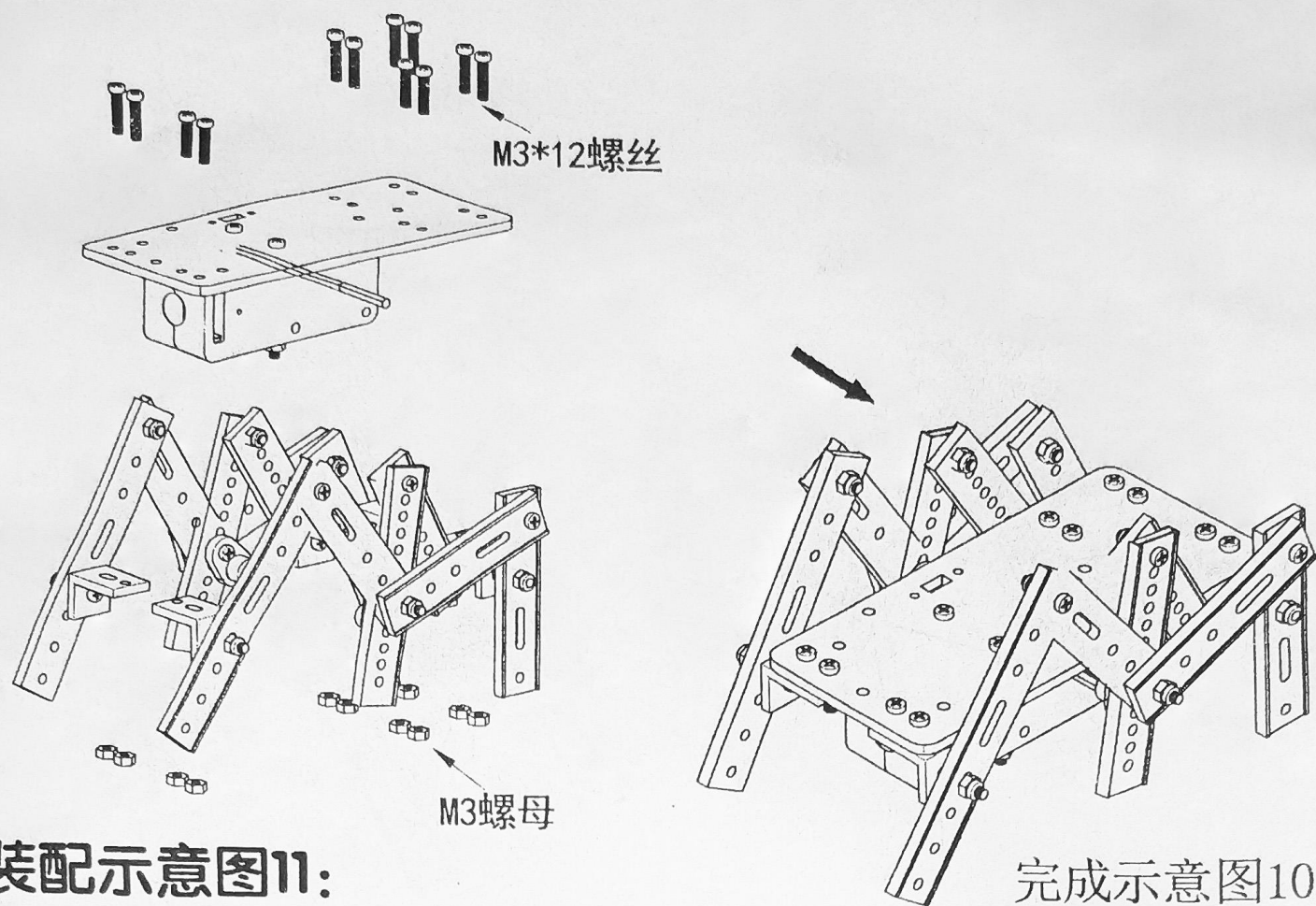
装配示意图10:
