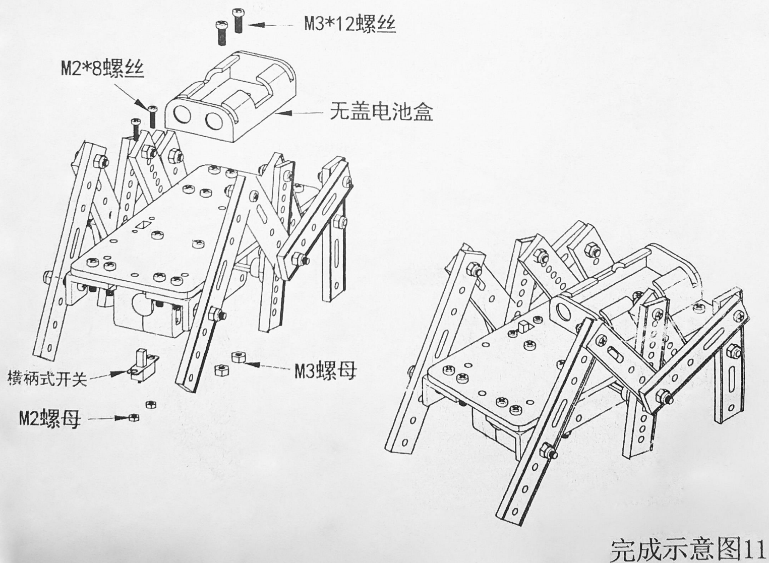
装配示意图11:
