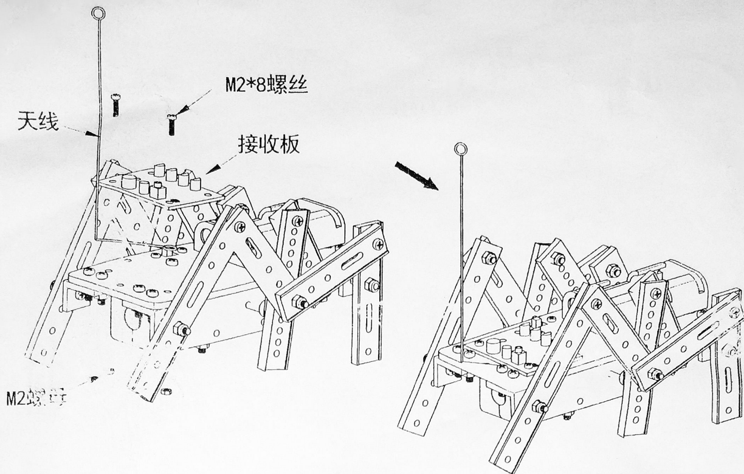
装配示意图13:
