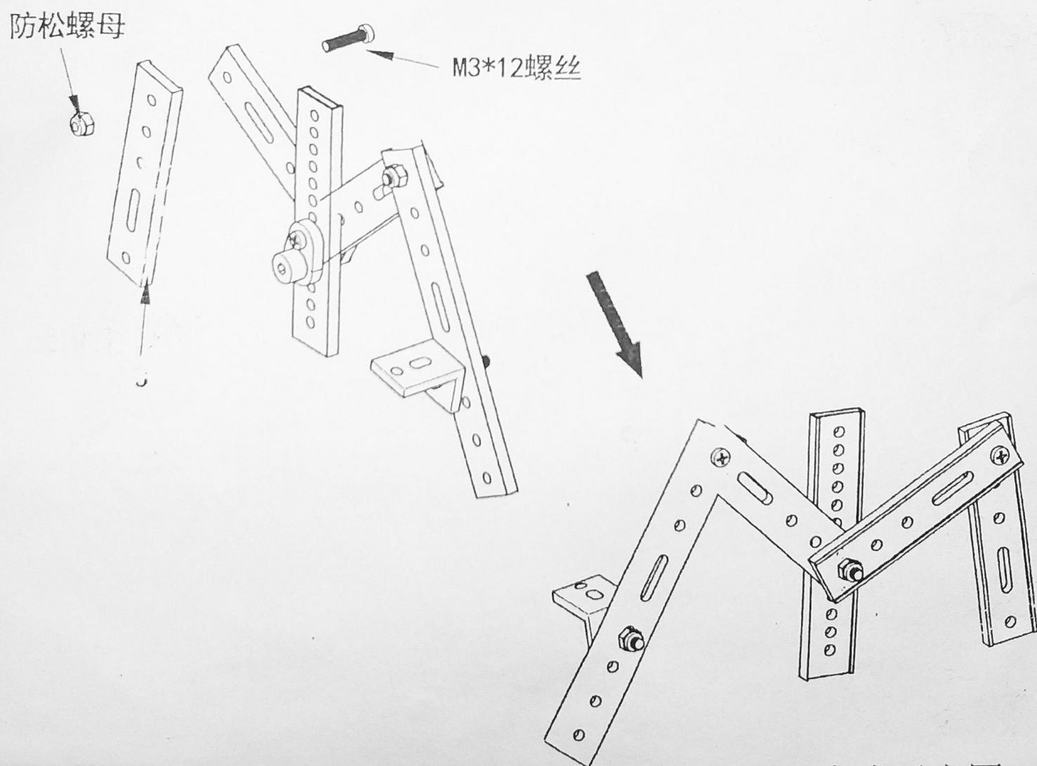
完成示意图05
