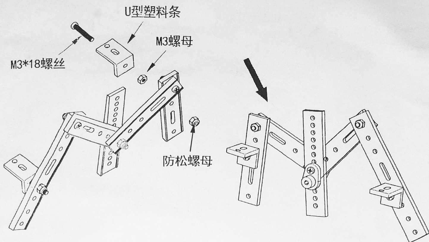
装配示意图07:
