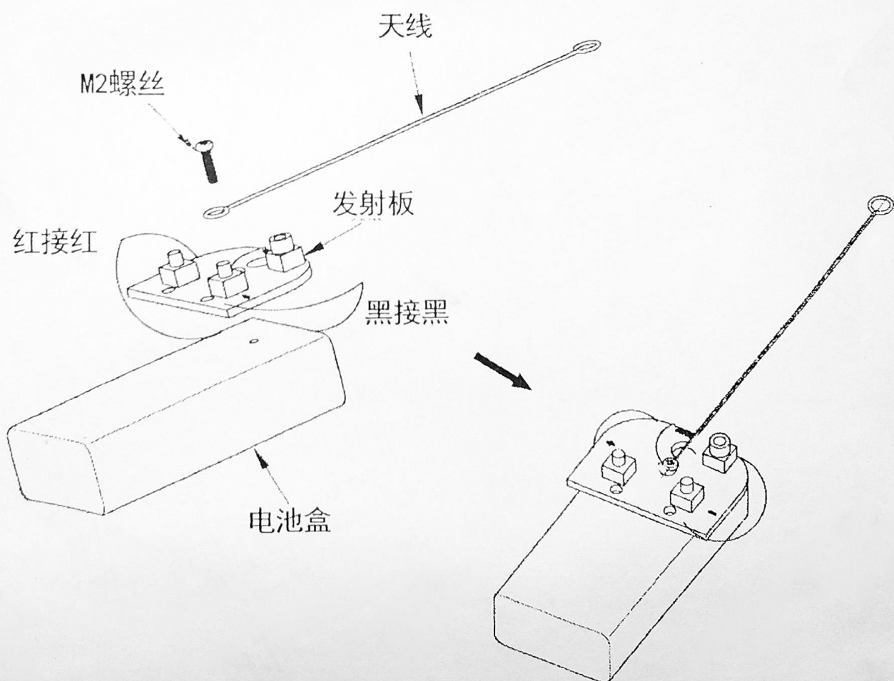
装配示意图13:
