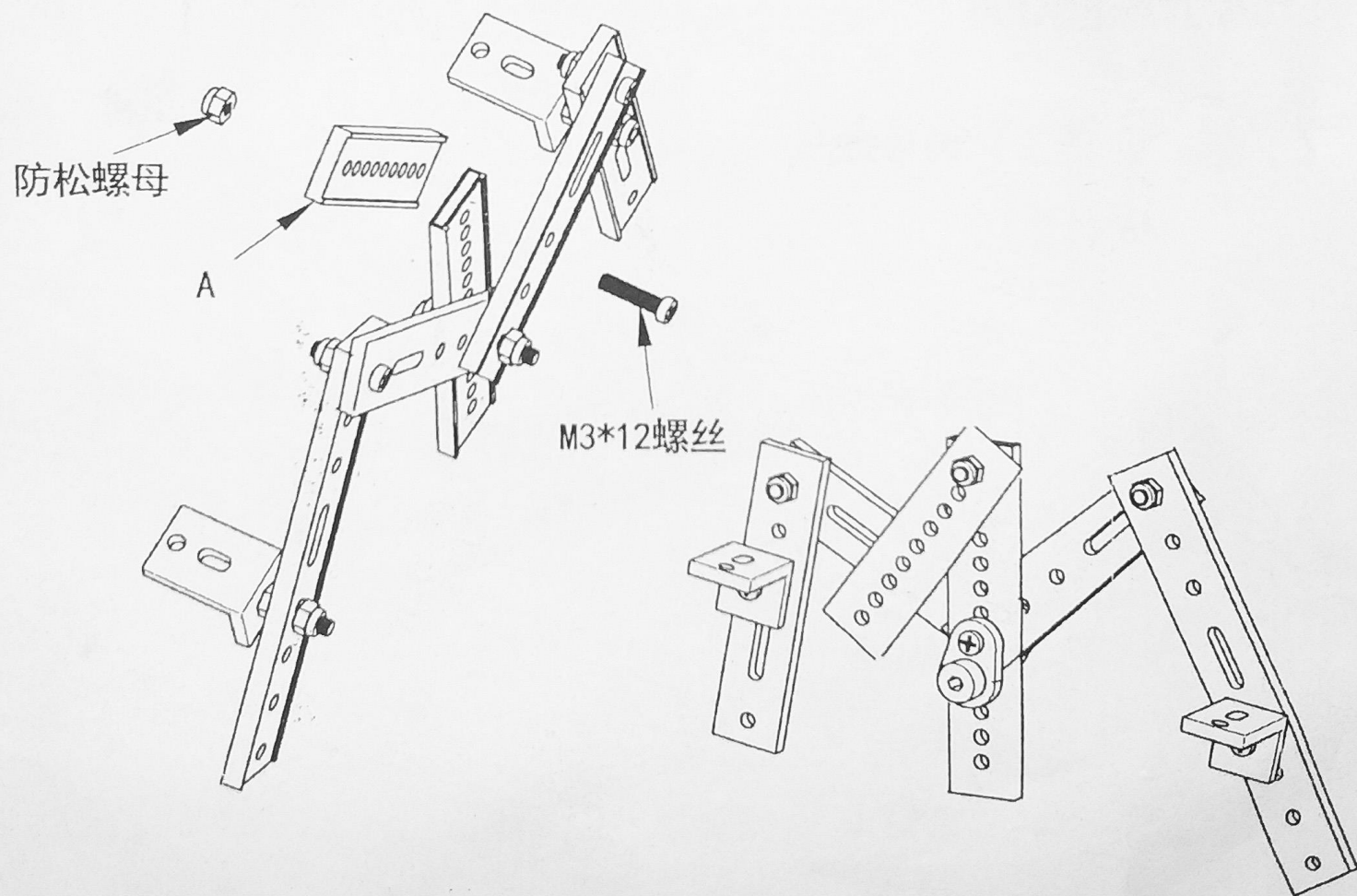
装配示意图07:
