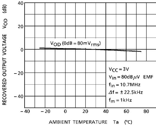
FM (IF) VOD - Ta
