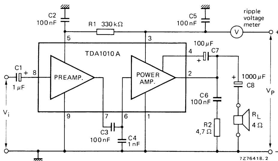
Fig.3 Test circuit.
