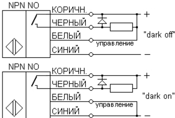
Работа выхода в режиме «dark on»
