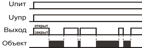
Работа выхода в режиме «dark off»
