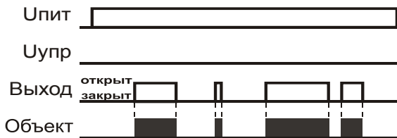
Работа выхода в режиме «dark on»
